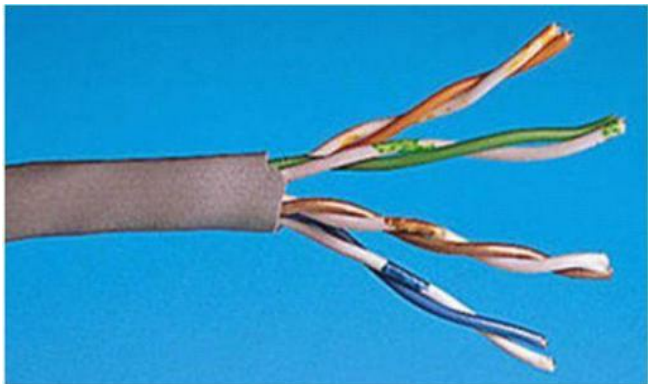
Figura 8.3 – Cabos de par trançado com quatro pares trançados (cada par é uma trança).
