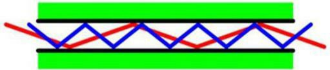
Figura 8.13 – Esquema de funcionamento da fibra multimodo.
