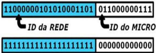
Figura 8.72 – Os 20 primeiros bits representam o ID da rede.
