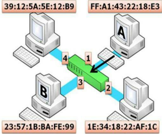
Figura 8.53 – Micro “A” envia um quadro ao switch.
