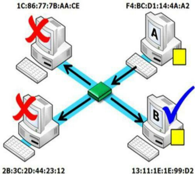
Figura 8.45 – Funcionamento da Ethernet sob a óptica dos endereços MAC.
