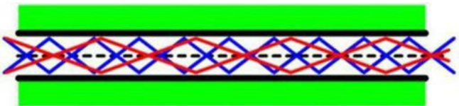
Figura 8.14 – Esquema de uma fibra óptica multimodo de índice degrau.
