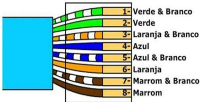
Figura 8.6 – Configuração T568-A.
