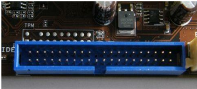
Figura 2.84 – Slot IDE.
