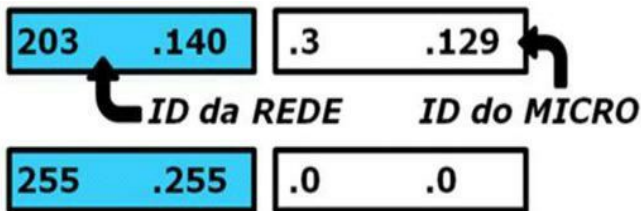
Figura 8.69 – Analisando o IP 203.140.3.129 na máscara 255.255.0.0 (classe B).
